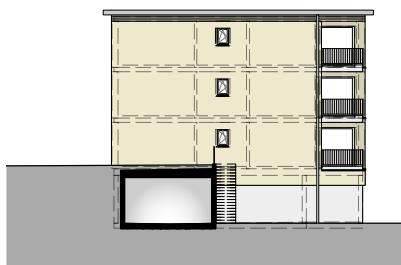
Lätternweg 21-27 Fassade Nord
