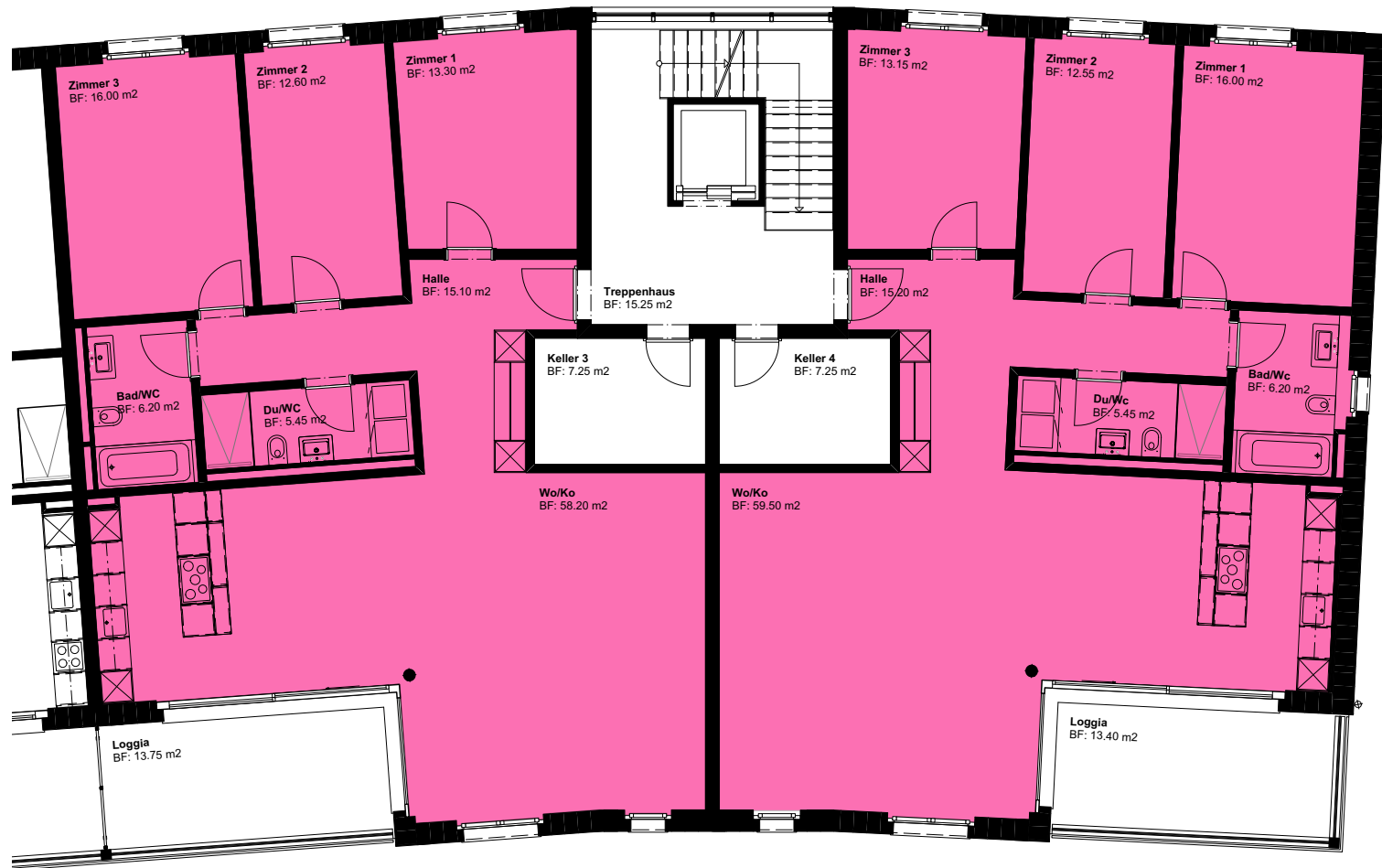
Lätternweg 45 Niveau 2-3 4.5 Zimmer-Wohnung BF: 126.85 m 2
